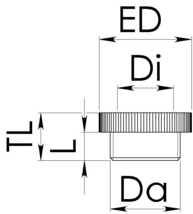
Maßzeichnung
