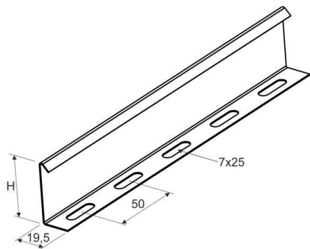
Maßzeichnung
