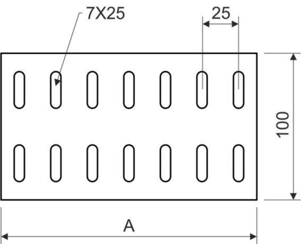
Maßzeichnung
