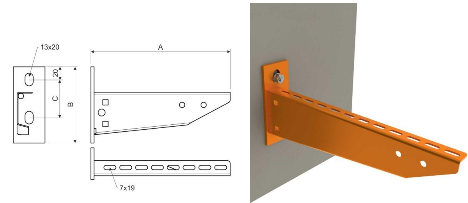
Maßzeichnung
