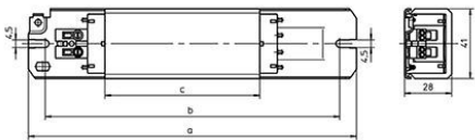
Maßzeichnung
