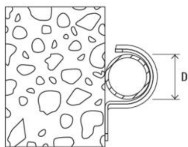
Strichzeichnung
