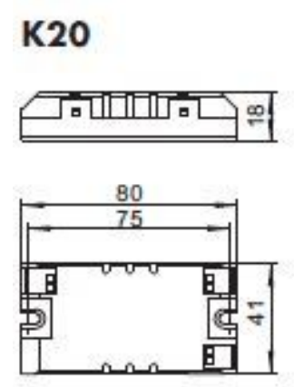
Maßzeichnung
