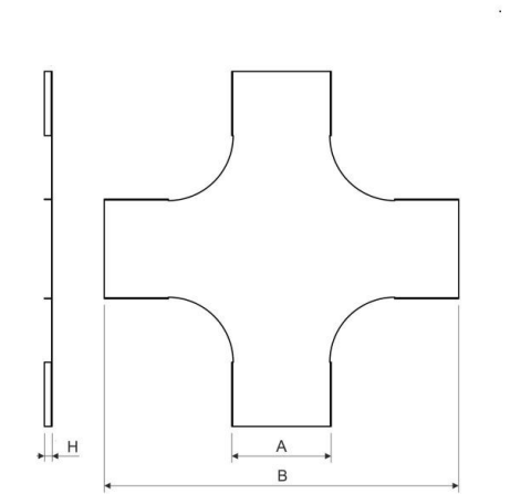
Maßzeichnung
