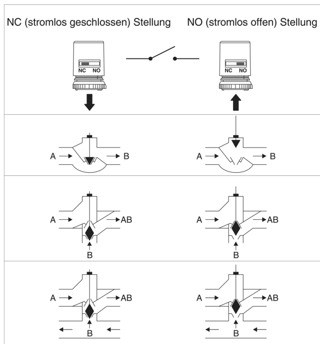
Abb. 6. Ventilfunktion
