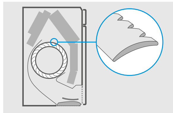
Neu gestalteter Ventilator mit noch niedrigeren Geräuschpegel und wirkungsvoller Schalldispersion
