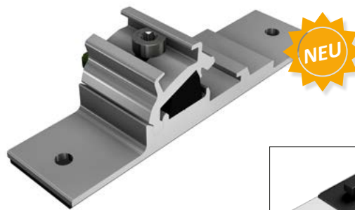
Mit vormontierten EPDM-Gummistreifen (UV-beständig)
