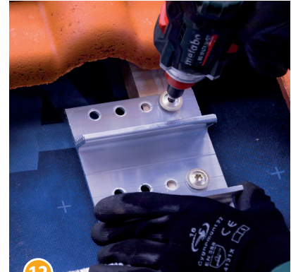
12 Fuß mit mind. 2 Holzschrauben (mind. 1 Stück pro horizontale Lochreihe, 10 Nm) am Dachsparren befestigen.
