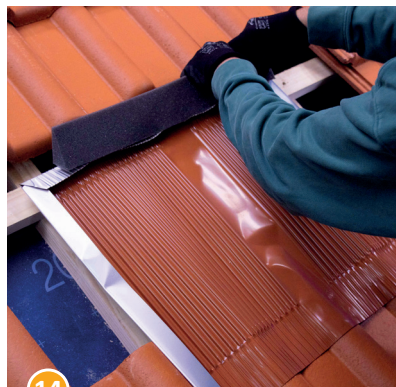
14 Schaumstoffkeil auf der hinteren Blechkantung der Beta-Platte festkleben.
