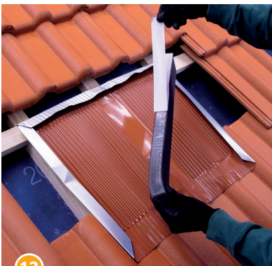
13 Schutzfolie des Klebestreifens auf der Unterseite des Schaumstoffkeils abziehen. Auf einen sauberen, staubfreien und trockenen Untergrund der zu beklebenden Fläche achten!
