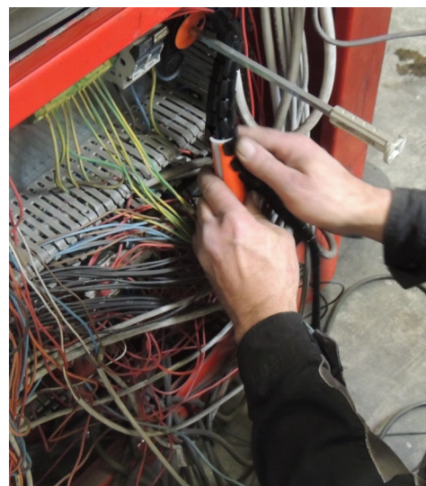
3 Die Schlauch mit einer Hand halten und den Spreizer gleiten lassen: die Kabeln werden durch den Schlauch "geschluckt".
