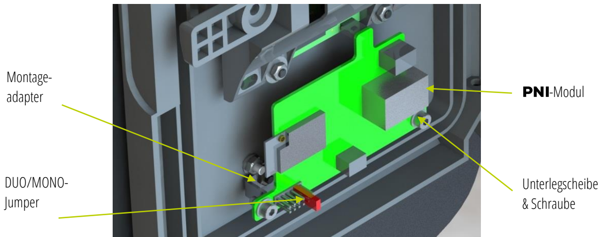
Abbildung 6 Montiertes Modul in ALPHA MONO
