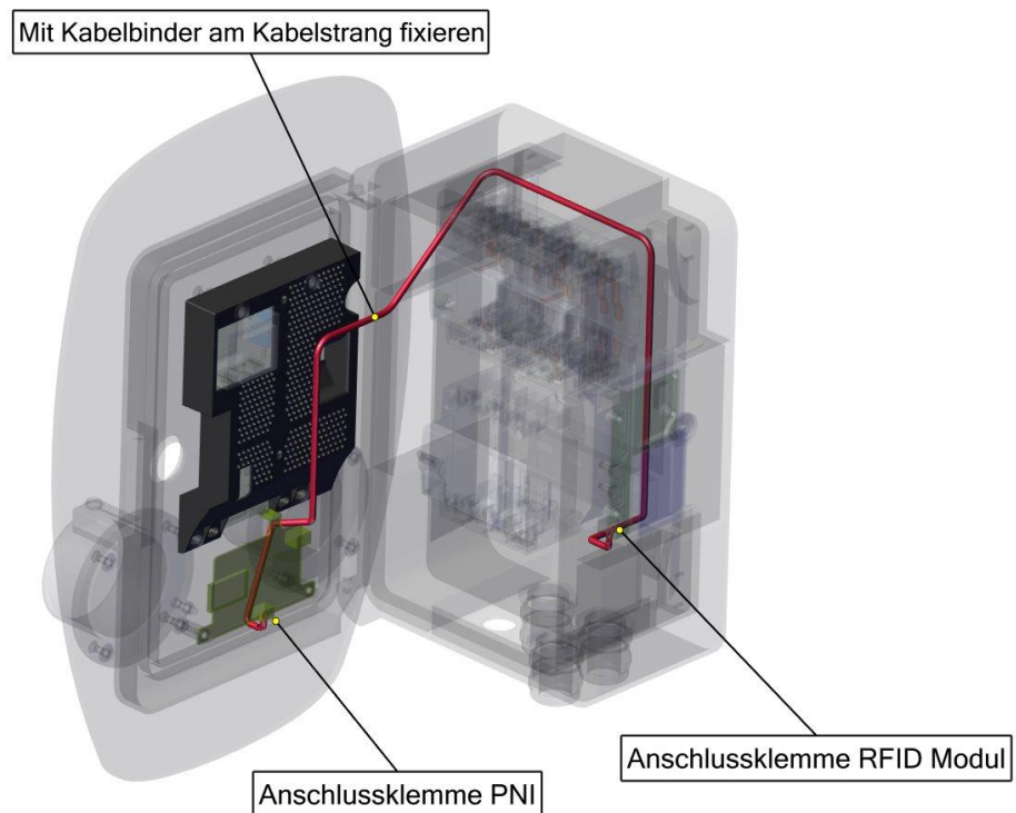
Abbildung 8 Montageempfehlung Modbus Leitung Wallbox Alpha
