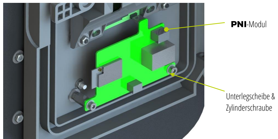
Abbildung 3 Montiertes Modul in ALPHA Doppellader
