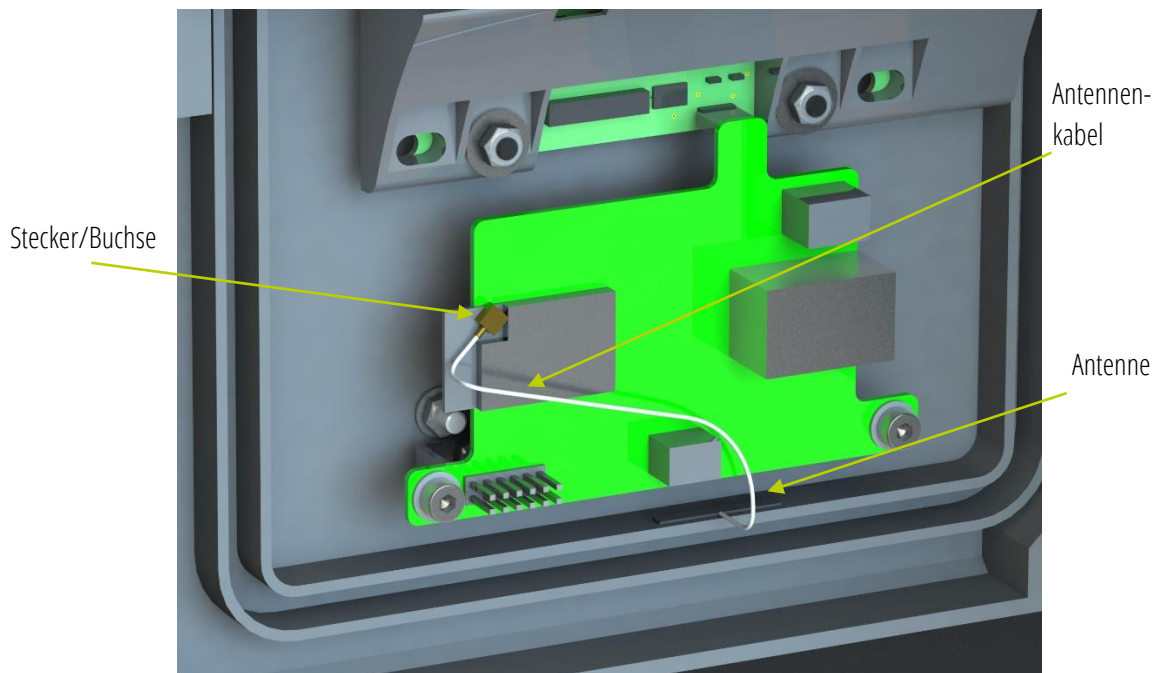
Abbildung 7 Montage der WLAN Antenne
