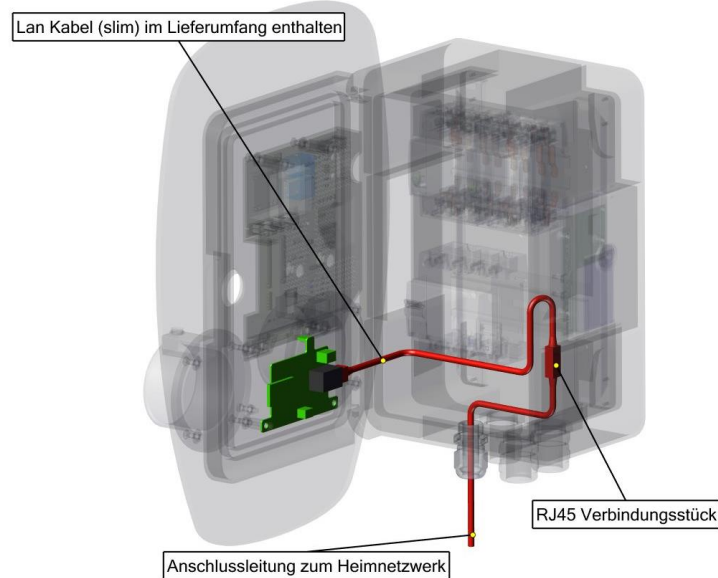
Abbildung 9 Empfehlung Verlegung Netzwerkleitung
