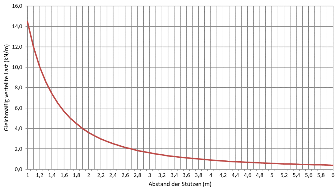
Zulässige Belastung KLWS 100/500 d=1,5mm (kN/m)
