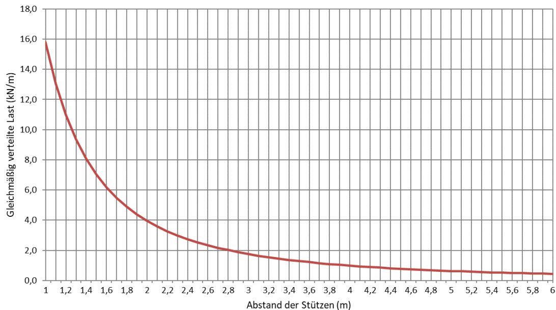
Zulässige Belastung KLWS 100/400 d=1,5mm (kN/m)
