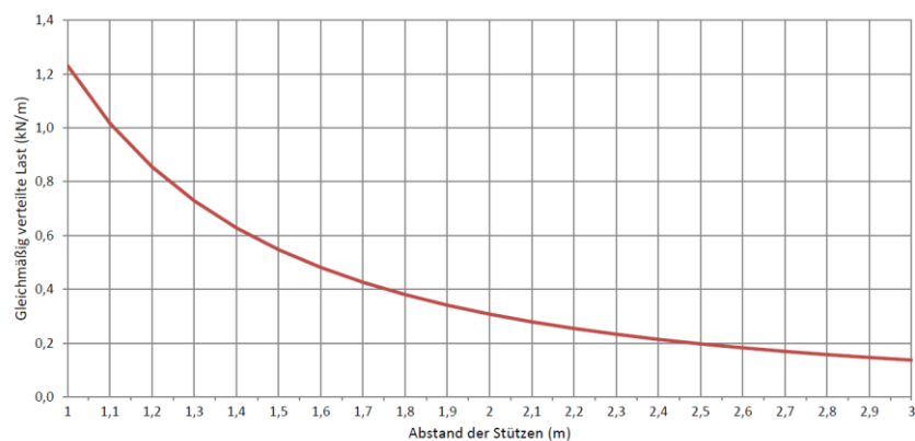
Zulässige Belastung KPK 60/100 d=0,6mm (kN/m)
