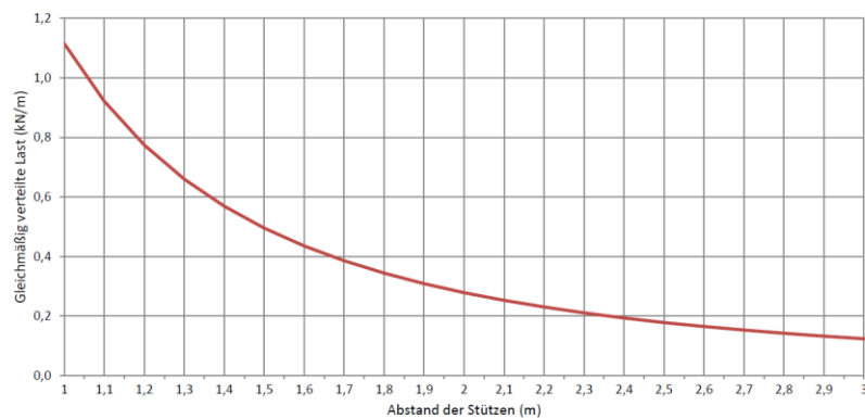
Zulässige Belastung KPK 40/100 d=0,6mm (kN/m)
