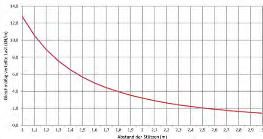
Zulässige Belastung KL 100/600 d=1,5mm (kN/m)
