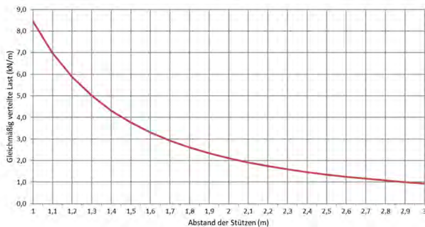
Zulässige Belastung KL 100/400 d=1,0mm (kN/m)
