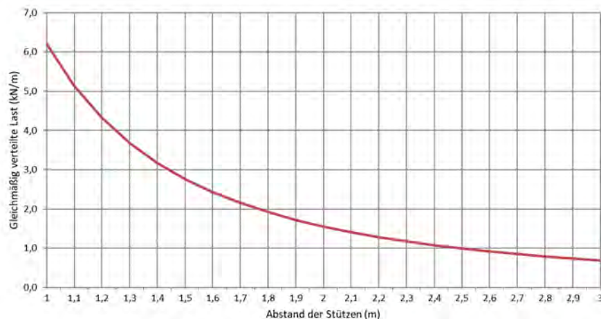
Zulässige Belastung KL 60/600 d=1,0mm (kN/m)
