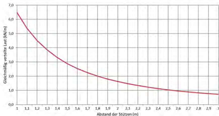
Zulässige Belastung KL 60/300 d=1,0mm (kN/m)
