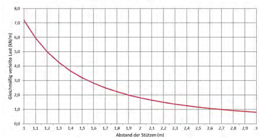
Zulässige Belastung KL 60/400 d=1,0mm (kN/m)
