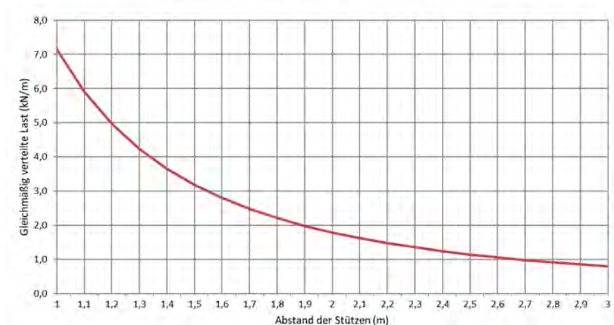
Zulässige Belastung KL 100/300 d=1,0mm (kN/m)
