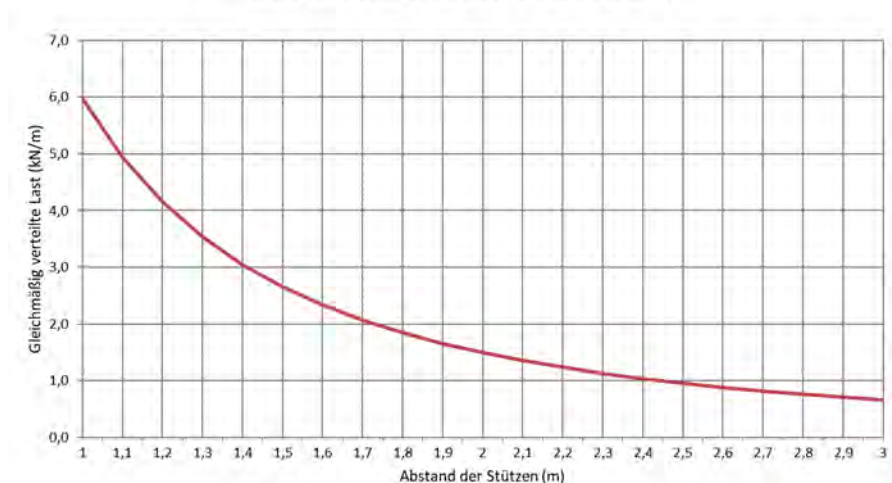
Zulässige Belastung KL 60/500 d=1,0mm (kN/m)
