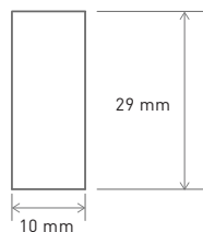
Profilhalterung:
