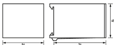
Maßzeichnung Sicherungssteckersätze DSE Do-13
