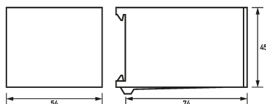
Maßzeichnung Sicherungssteckersätze DSE Do-o6
