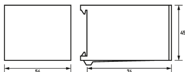
Maßzeichnung Sicherungssteckersätze DSE Do-02
