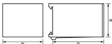
Maßzeichnung Sicherungssteckersätze DSE Do-01
