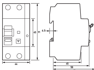
Maßzeichnung FI-/LS-Kombinationen DRCBO 4 C25/0,30/1N-B+
