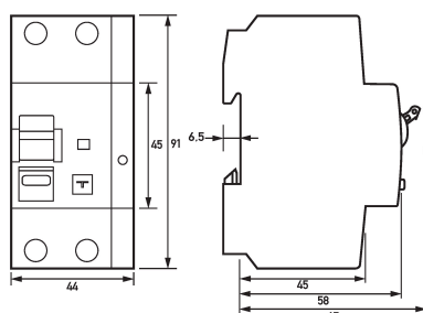
Maßzeichnung FI-/LS-Kombinationen DRCBO 4 C16/0,30/1N-B+
