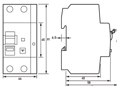
Maßzeichnung FI-/LS-Kombinationen DRCBO 4 B32/0,30/1N-B+
