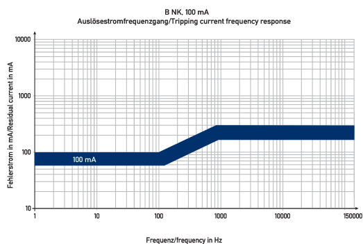
Diagramme FI-/LS-Kombinationen DRCBO 4 C16/0,10/1N-B NK
