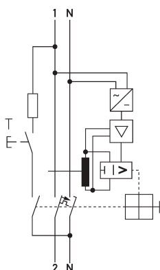
Schaltungsbeispiel FI-/LS-Kombinationen DRCBO 4 B32/0,10/1N-B NK
