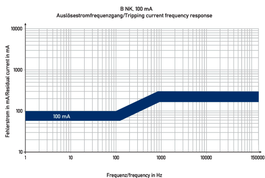
Diagramme FI-/LS-Kombinationen DRCBO 4 B32/0,10/1N-B NK
