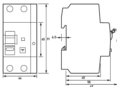
Maßzeichnung FI-/LS-Kombinationen DRCBO 4 B32/0,10/1N-B NK
