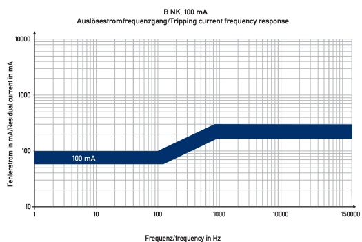
Diagramme FI-/LS-Kombinationen DRCBO 4 B25/0,10/1N-B NK
