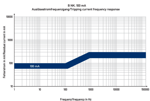
Diagramme FI-/LS-Kombinationen DRCBO 4 B13/0,10/1N-B NK
