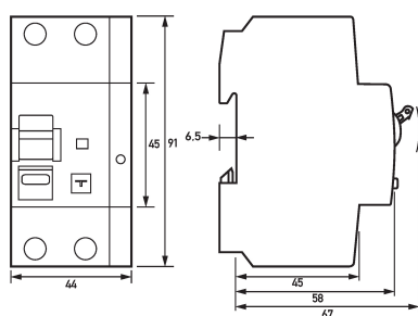
Maßzeichnung FI-/LS-Kombinationen DRCBO 4 B13/0,10/1N-B NK
