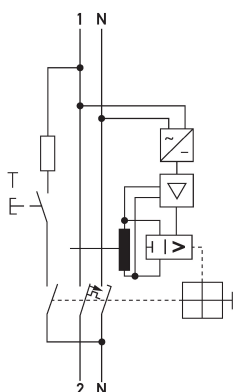
Schaltungsbeispiel FI-/LS-Kombinationen DRCBO 4 Bo6/o,10/1N-B NK
