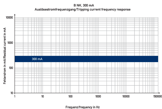
Diagramme FI-/LS-Kombinationen DRCBO 4 C13/0,30/1N-B NK
