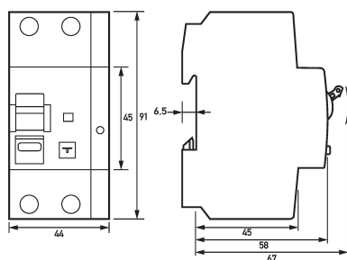
Maßzeichnung FI-/LS-Kombinationen DRCBO 4 C10/0,30/1N-B NK
