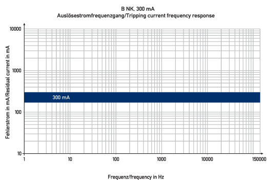
Diagramme FI-/LS-Kombinationen DRCBO 4 C10/0,30/1N-B NK
