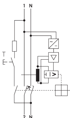
Schaltungsbeispiel FI-/LS-Kombinationen DRCBO 4 Co6/o,03/1N-B NK
