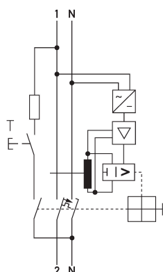
Schaltungsbeispiel FI-/LS-Kombinationen DRCBO 4 C10/0,10/1N-B SK
