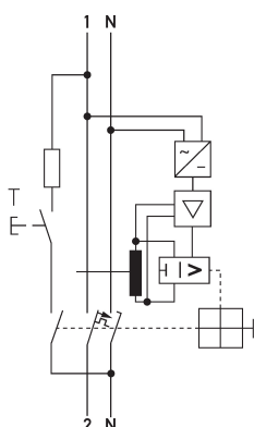
Schaltungsbeispiel FI-/LS-Kombinationen DRCBO 4 C32/0,30/1N-B SK
