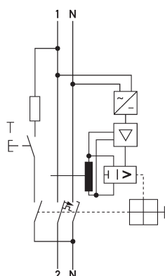
Schaltungsbeispiel FI-/LS-Kombinationen DRCBO 4 C20/0,30/1N-B SK
