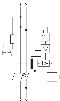
Schaltungsbeispiel FI-/LS-Kombinationen DRCBO 4 C13/0,30/1N-B SK
