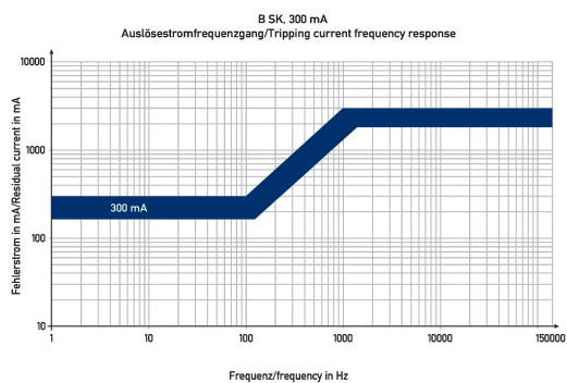
Diagramme FI-/LS-Kombinationen DRCBO 4 C13/0,30/1N-B SK
