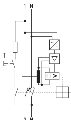
Schaltungsbeispiel FI-/LS-Kombinationen DRCBO 4 C10/0,30/1N-B SK
