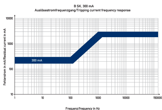
Diagramme FI-/LS-Kombinationen DRCBO 4 C10/0,30/1N-B SK
