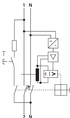
Schaltungsbeispiel FI-/LS-Kombinationen DRCBO 4 B16/o,30/1N-B SK
