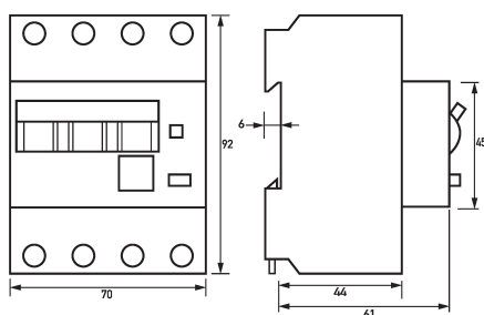
Maßzeichnung FI-/LS-Kombinationen DRCBO 4 C20/0,03/3N-F
