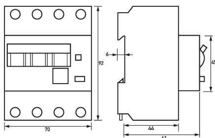
Maßzeichnung FI-/LS-Kombinationen DRCBO 4 B20/0,03/3N-F
