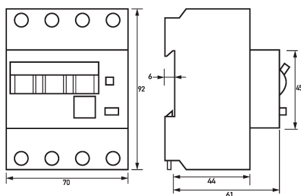
Maßzeichnung FI-/LS-Kombinationen DRCBO 4 Bo6/0,03/3N-F
